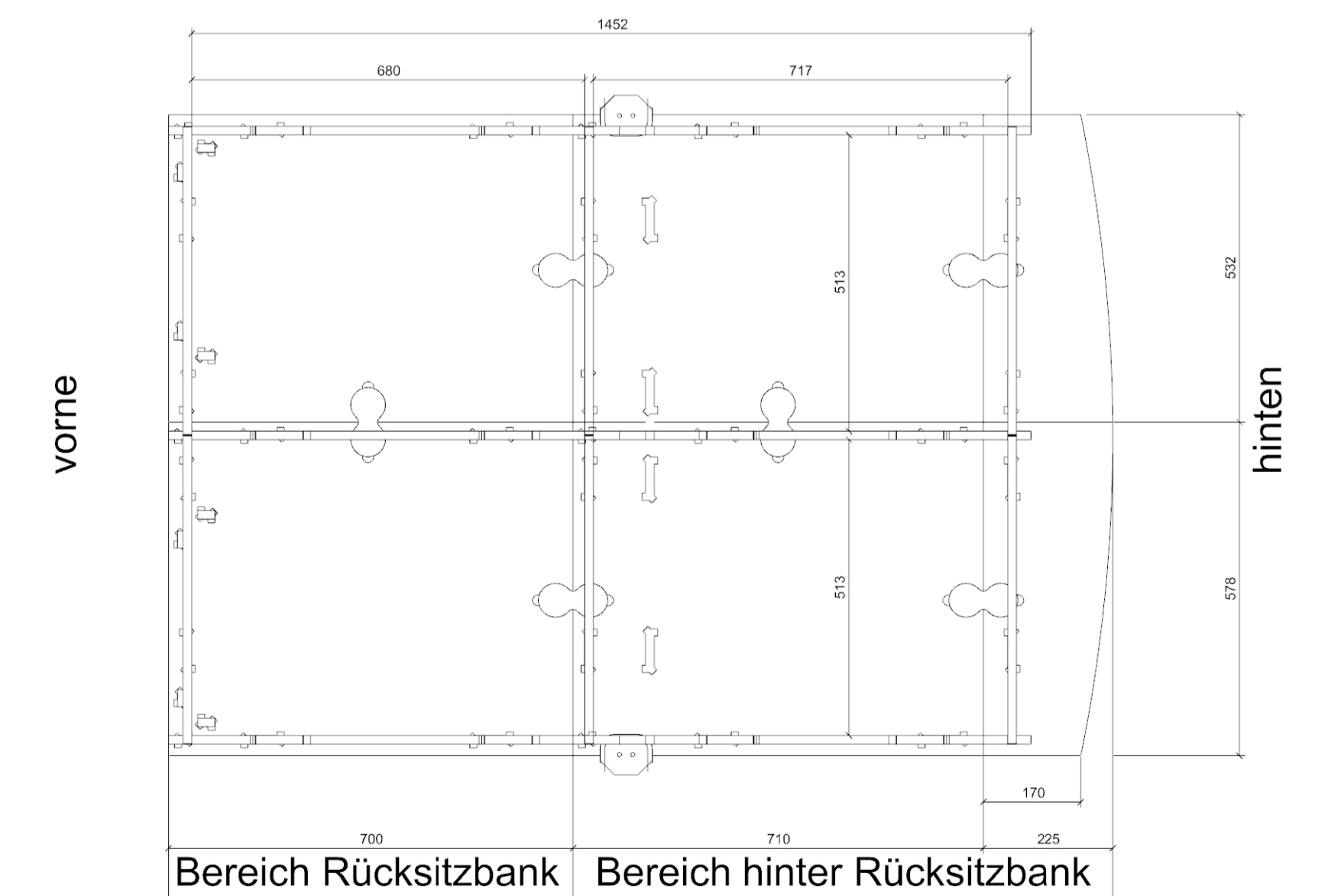
Ansicht oben
