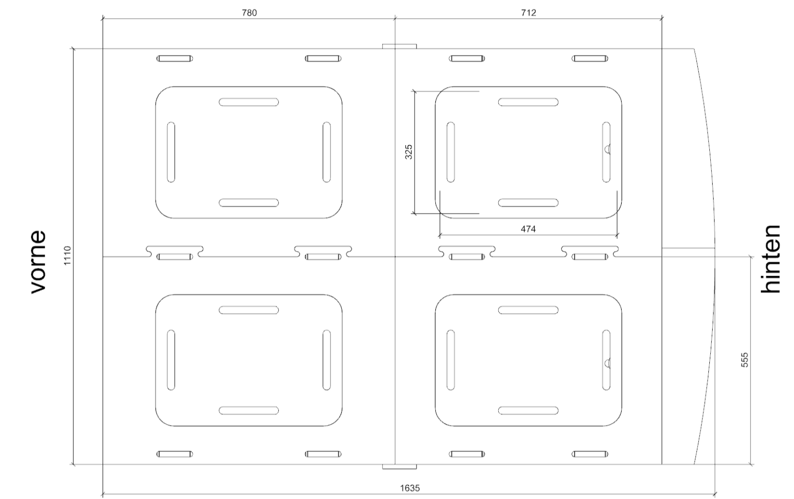
Ansicht oben
